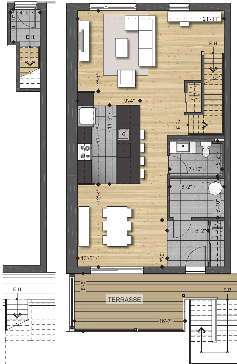
NIVEAU 1 COUR INTÉRIEURE
